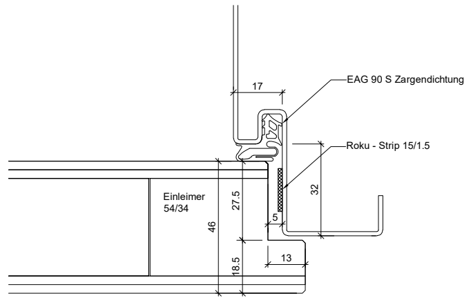
Umfassungszarge UD
