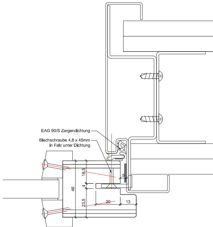
A-A Oberteil
