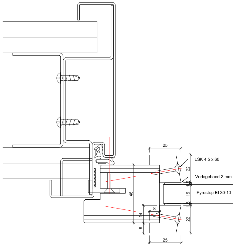
A-A Oberteil
