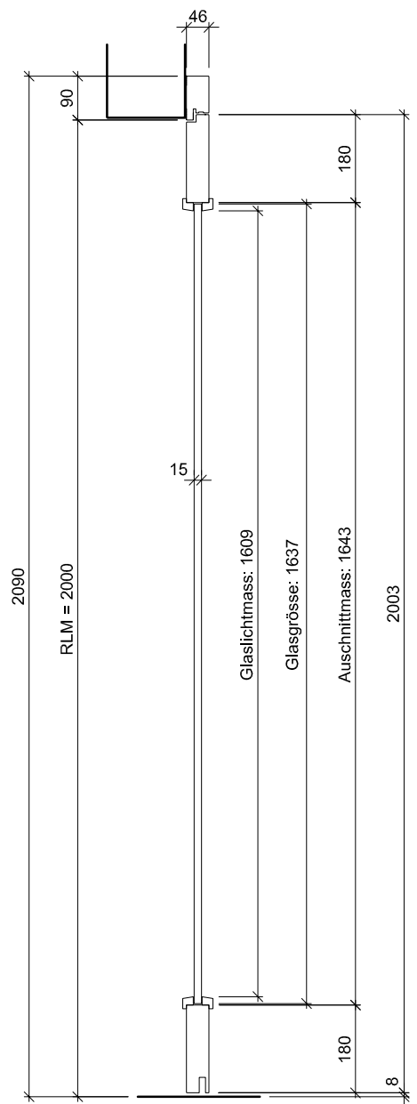
B-B
