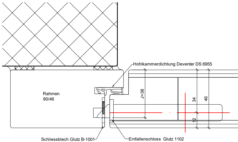
A-A Detail Schloss
