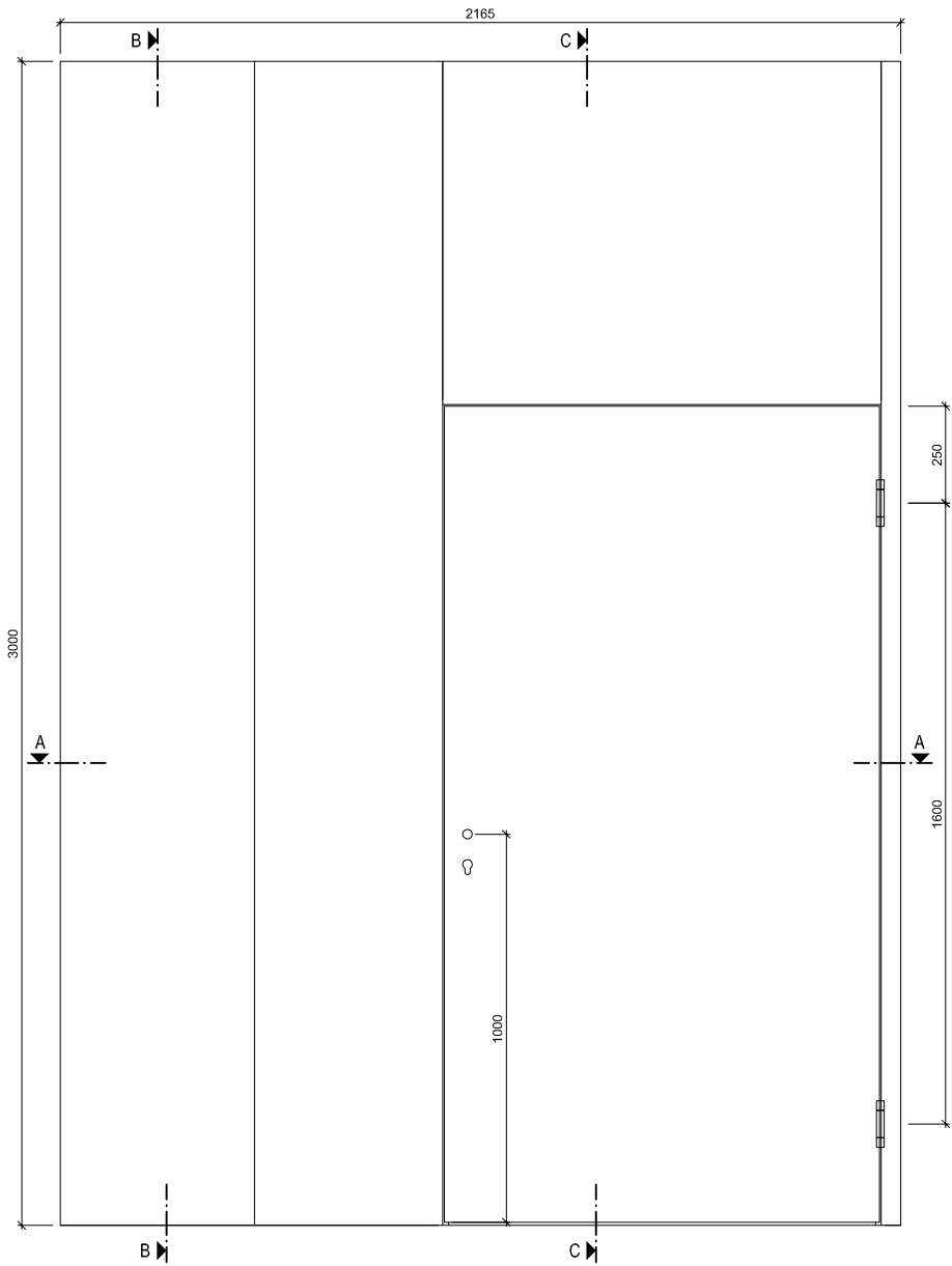
Ansicht
