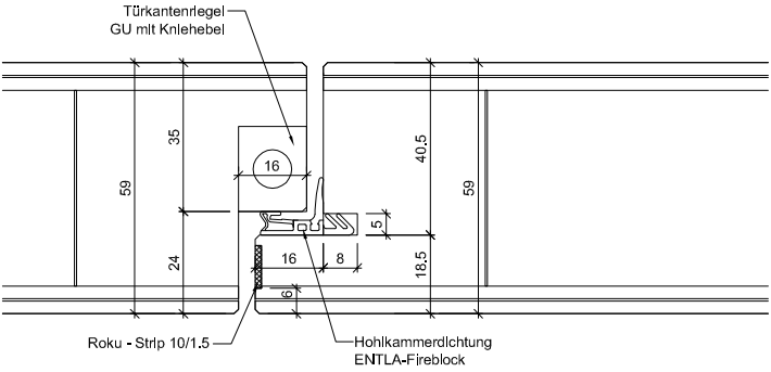
A-A Detail Kantenriegel oben
