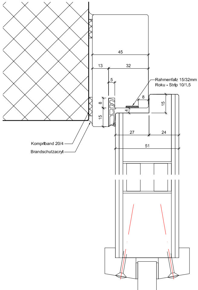
A-A Detail Schloss
