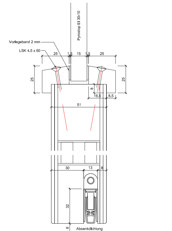
B-B Detail unten
