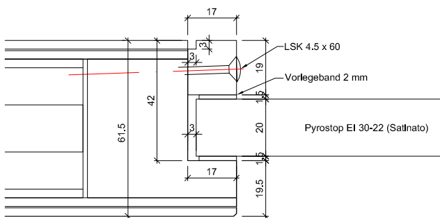
Ausschnitt gefälzt, Glasleisten stumpf
