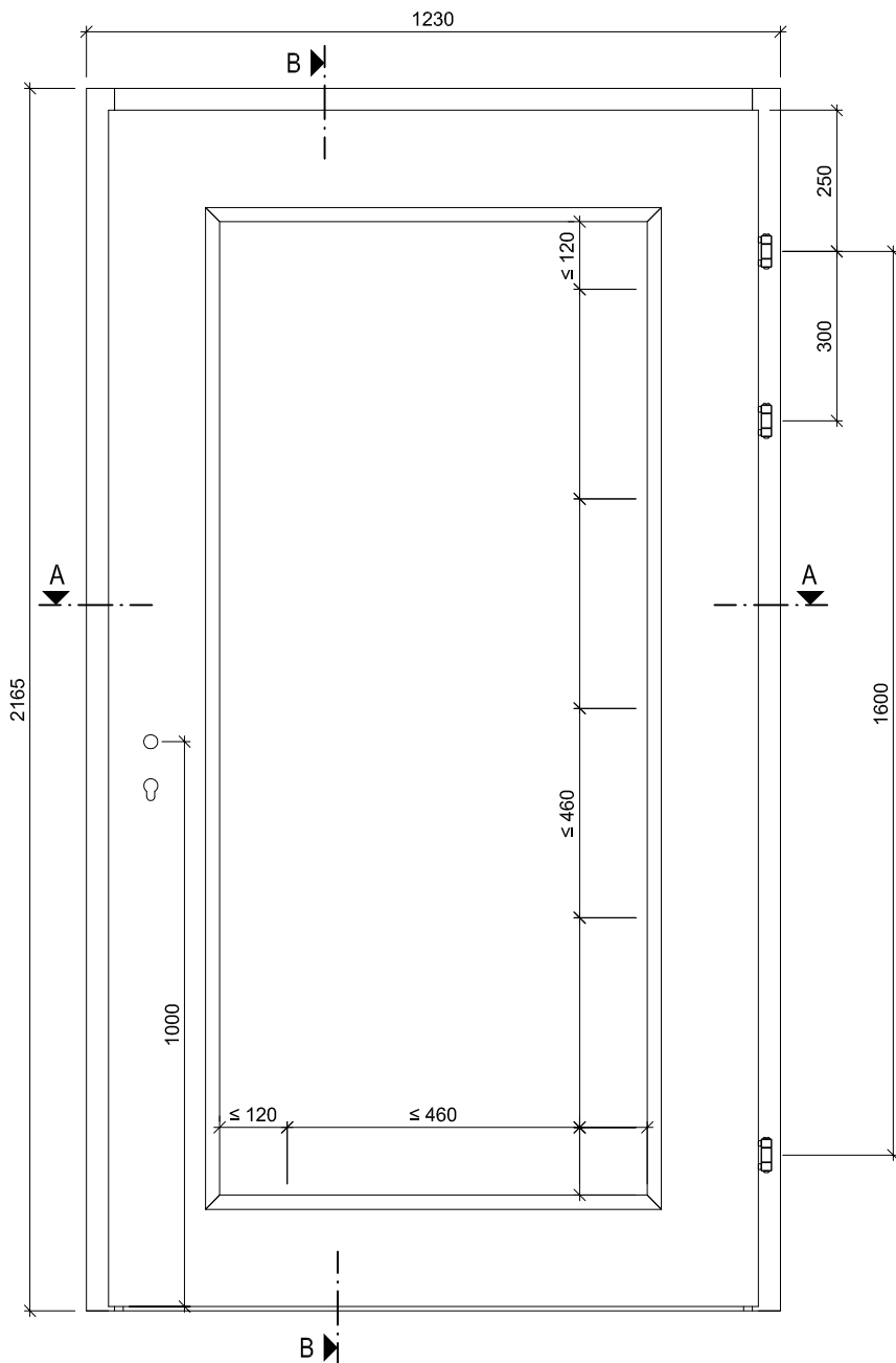
Ansicht
