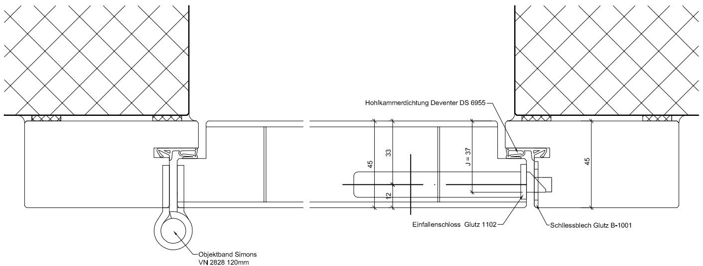
Detail A-A
