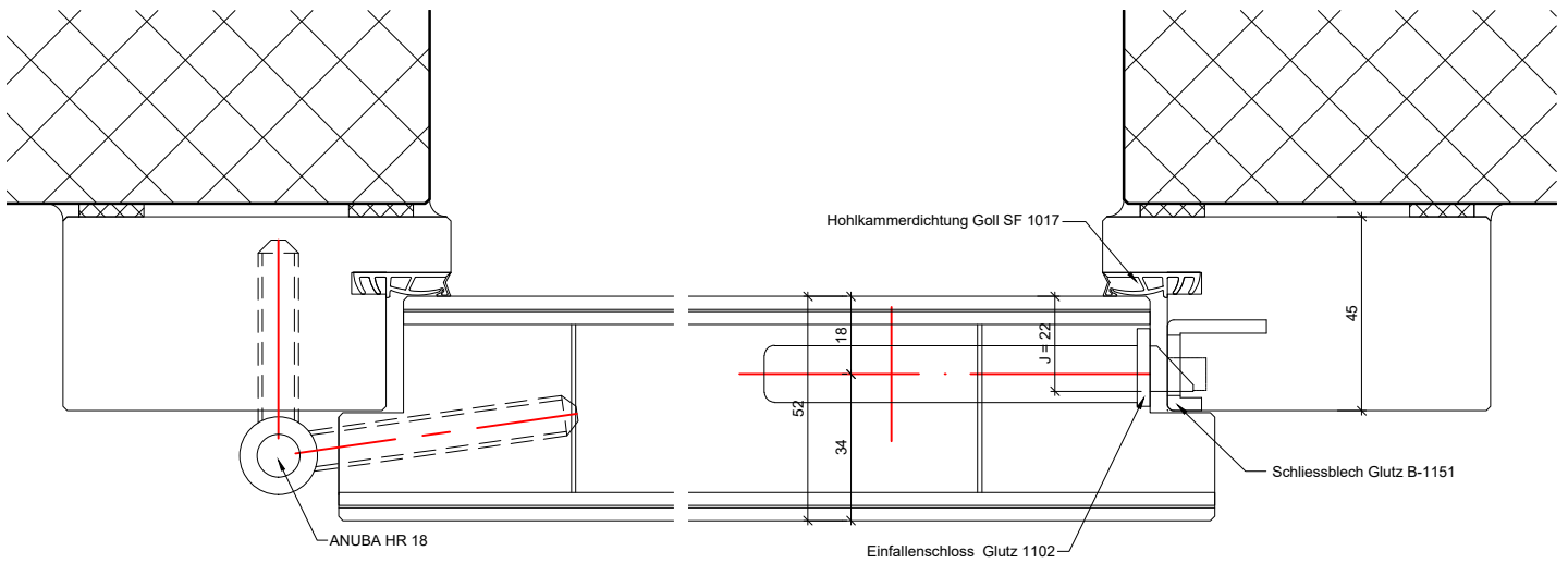
Detail A-A
