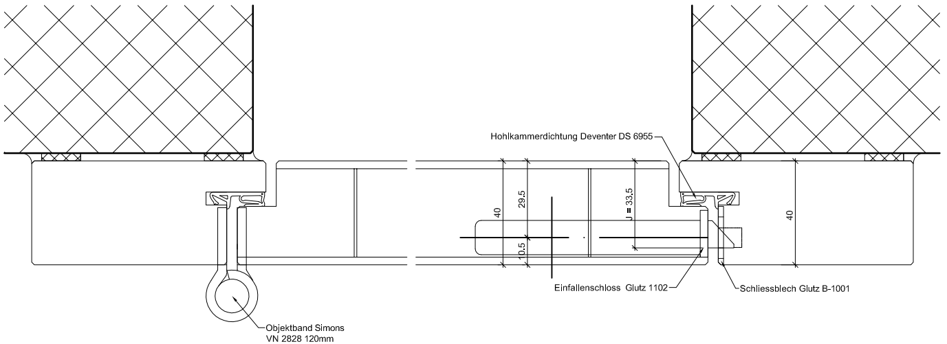
Detail A-A
