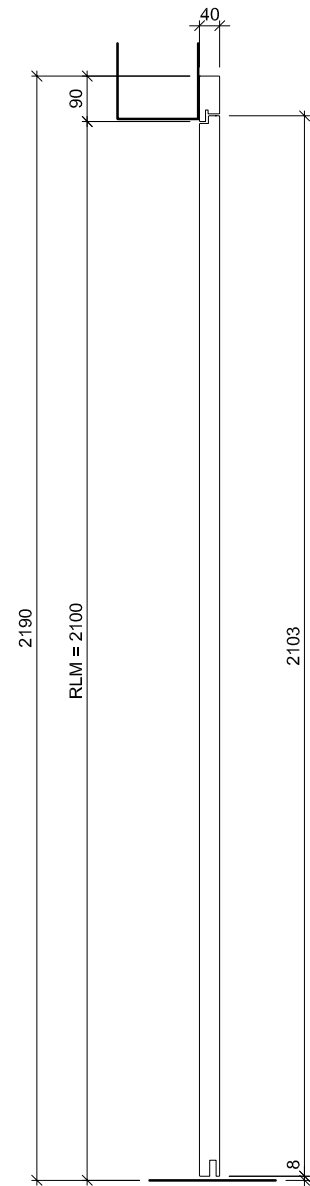
B-B
