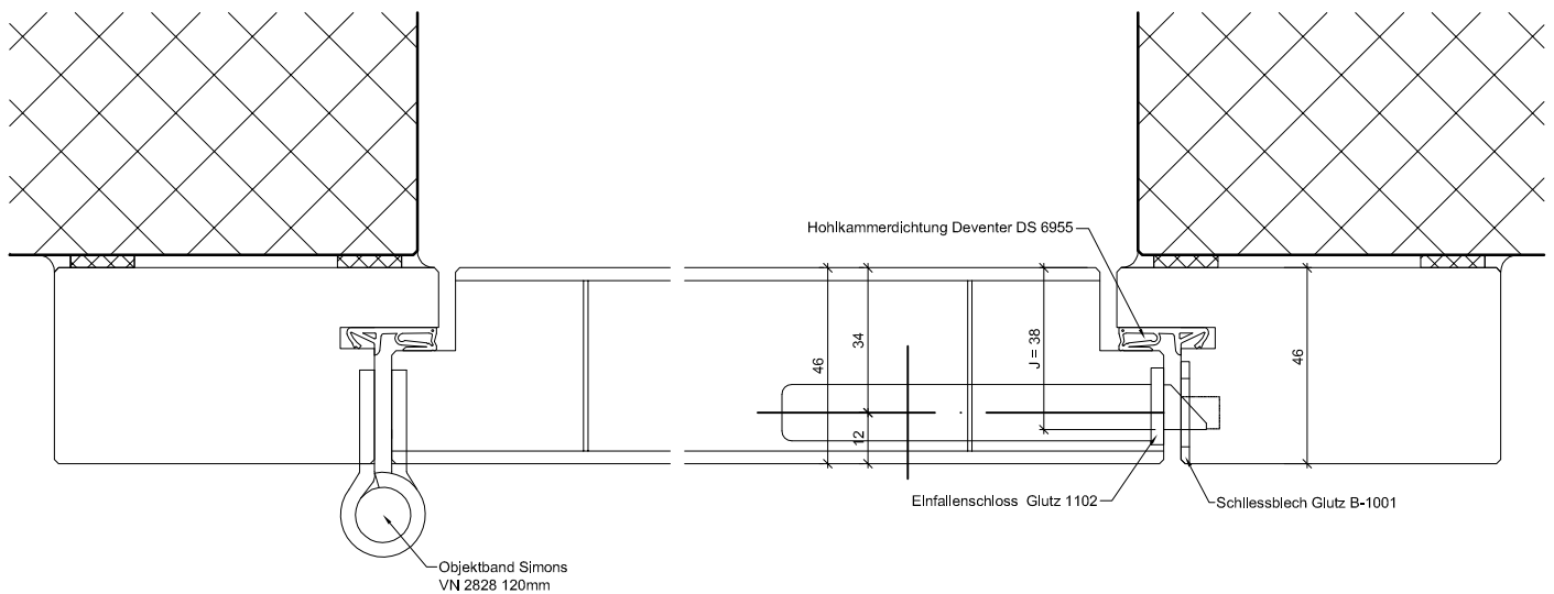
Detail A-A
