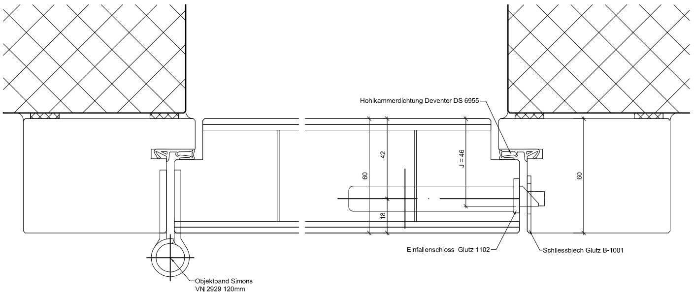
Detail A-A
