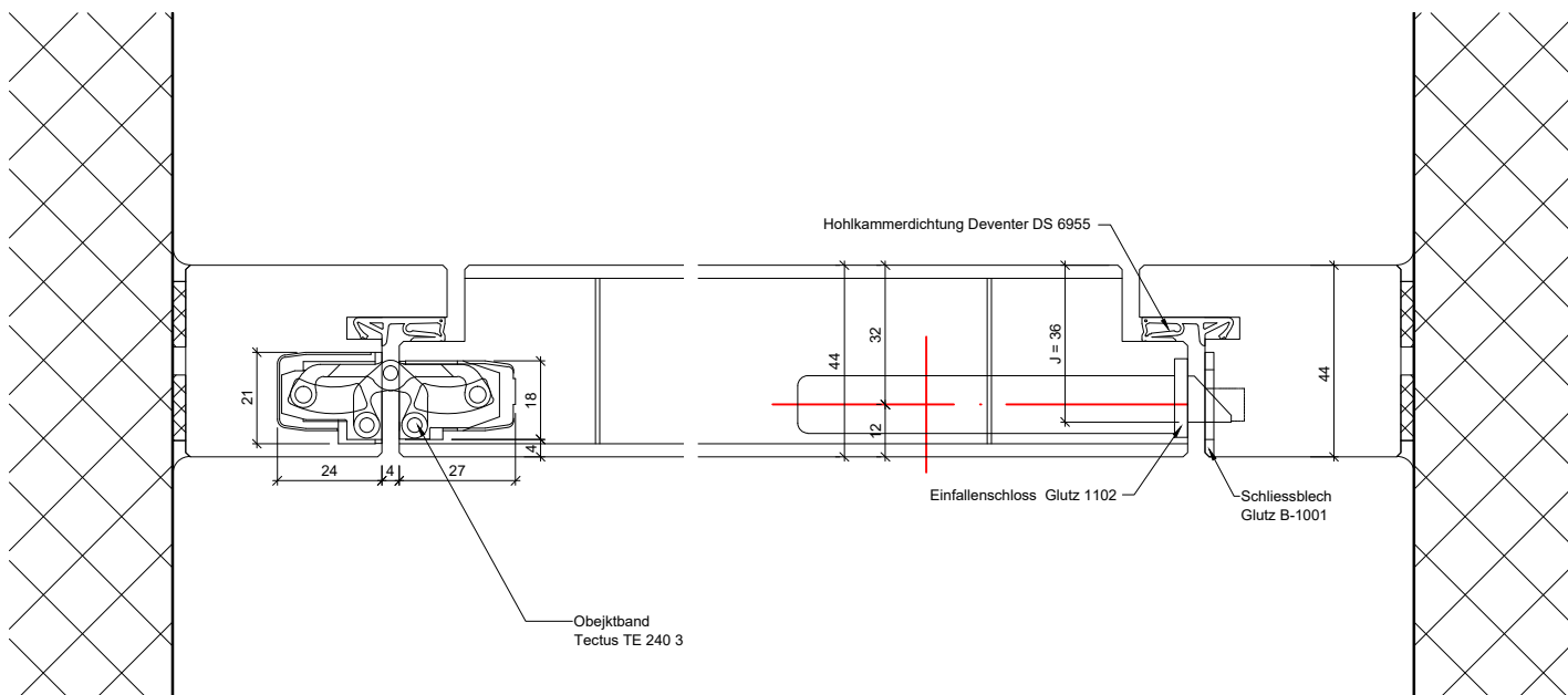
Detail A-A
