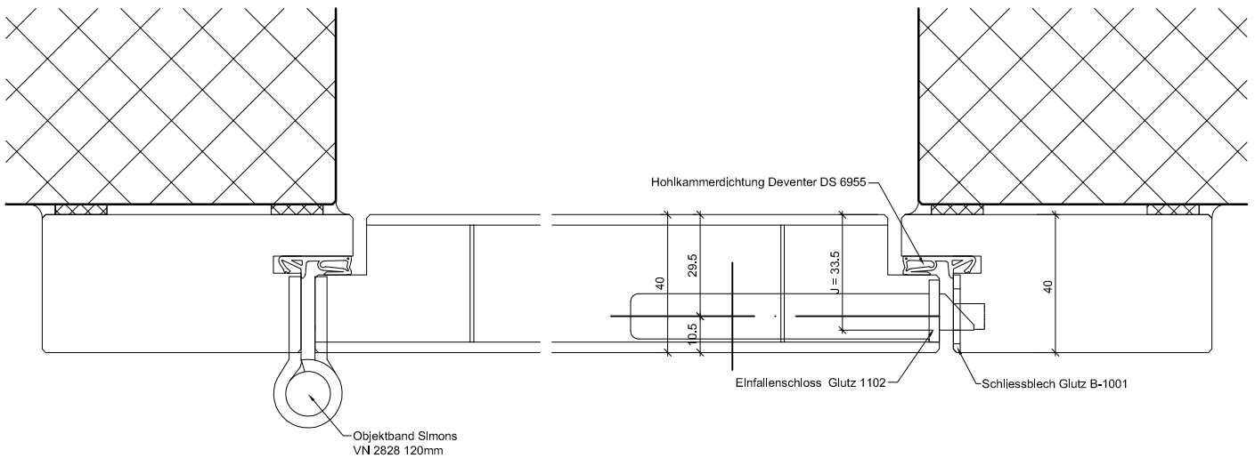
Detail A-A
