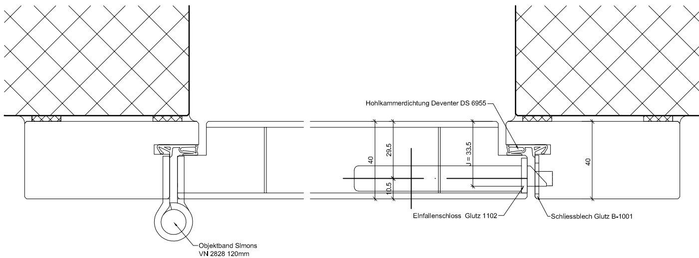
Detail A-A
