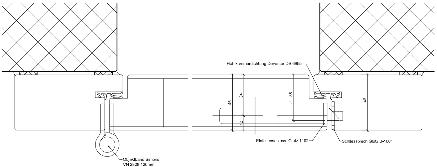
Detail A-A
