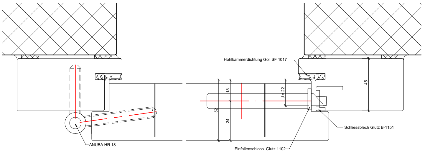
Detail A-A
